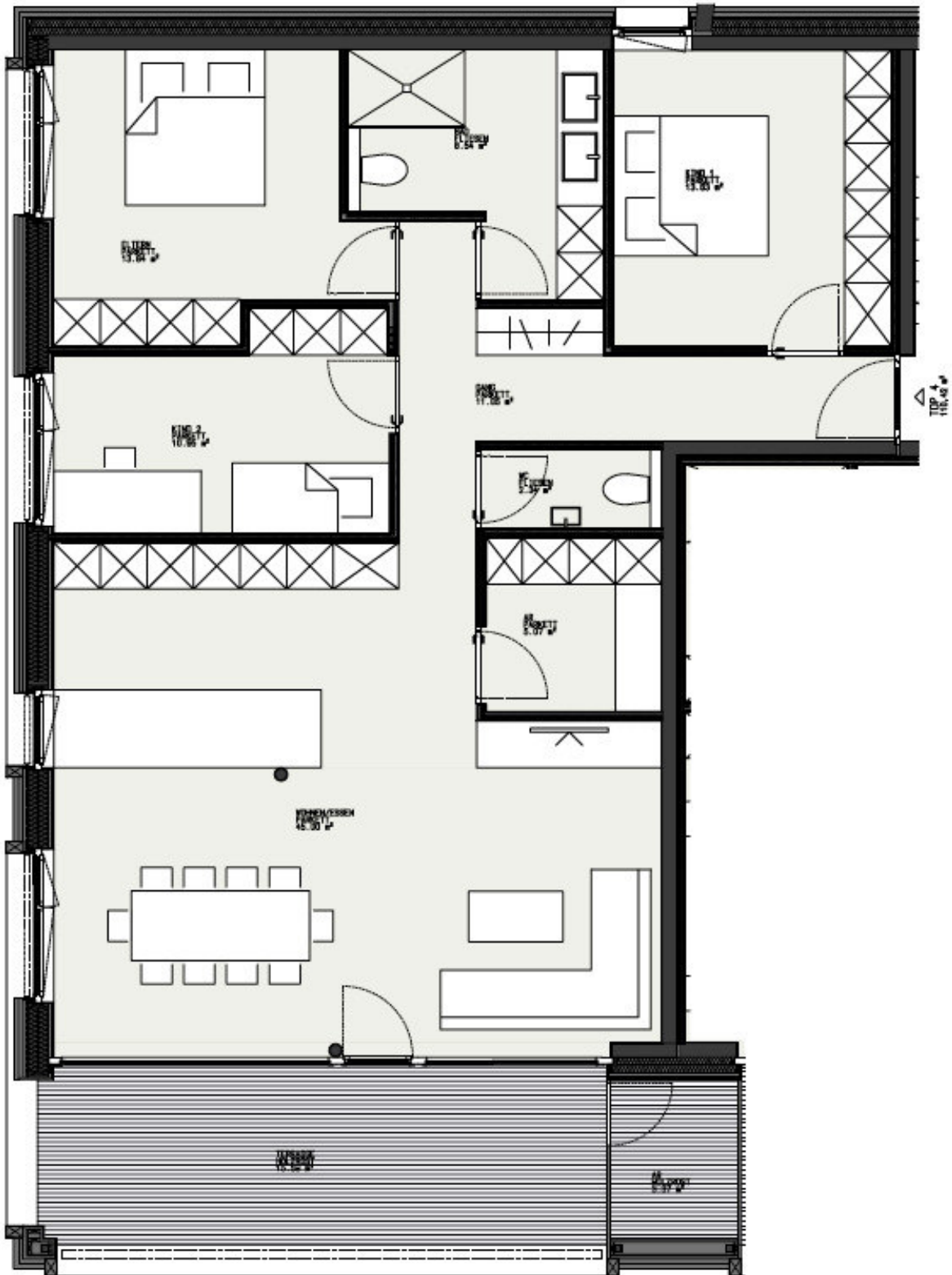
Grundrissplan
